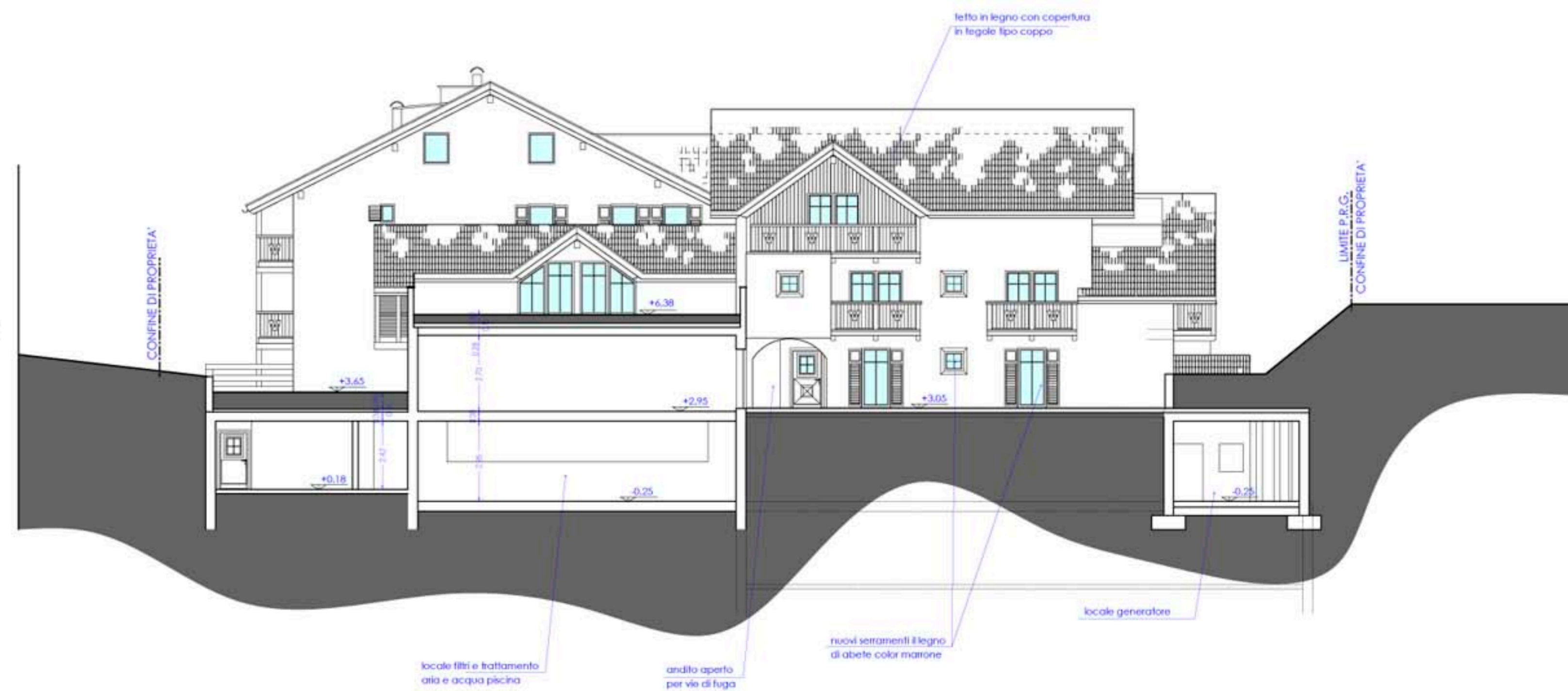
PROSPETTO OVEST
