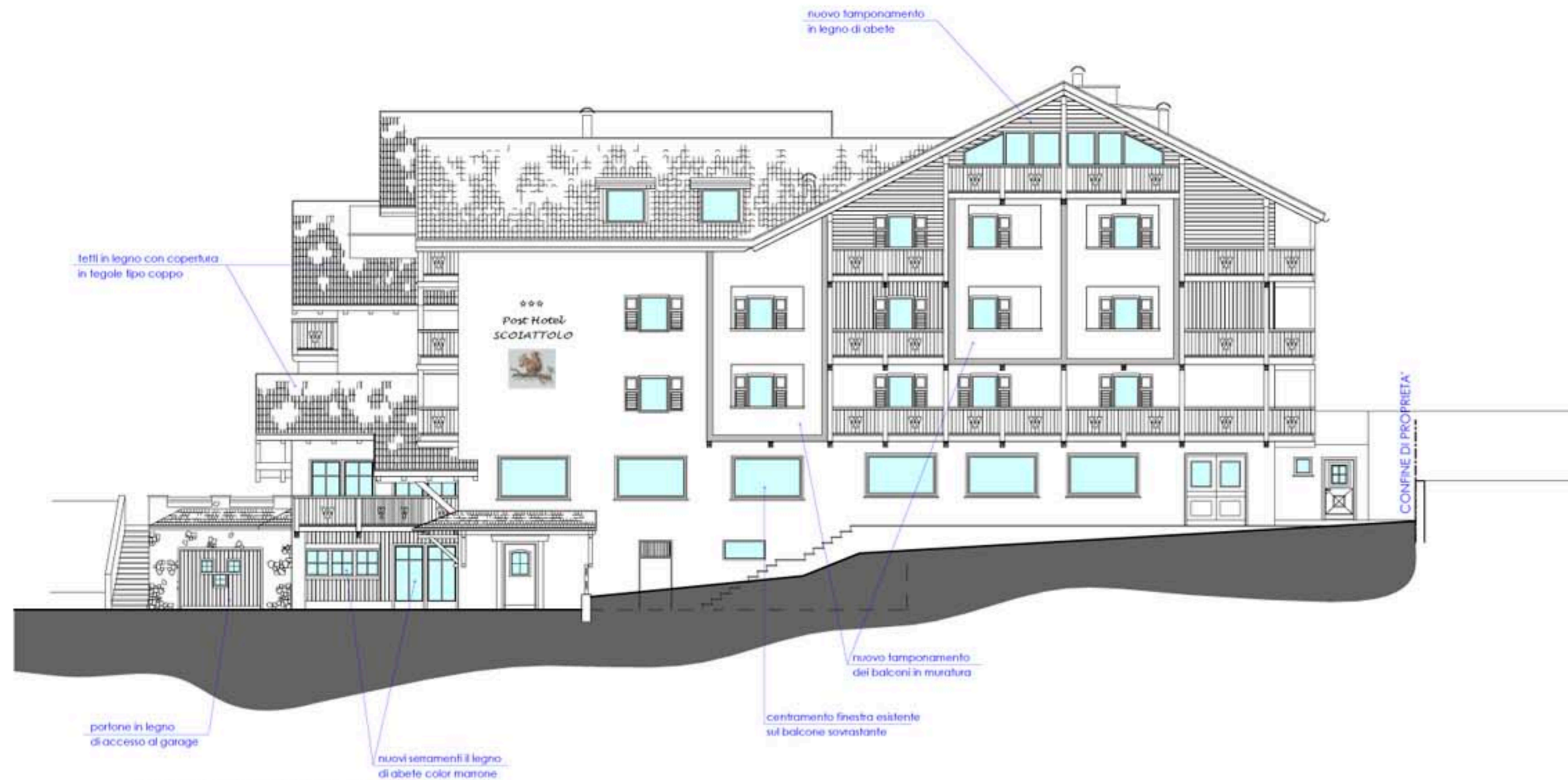
PROSPETTO SUD
