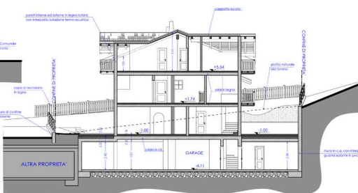
SEZIONE B-B
