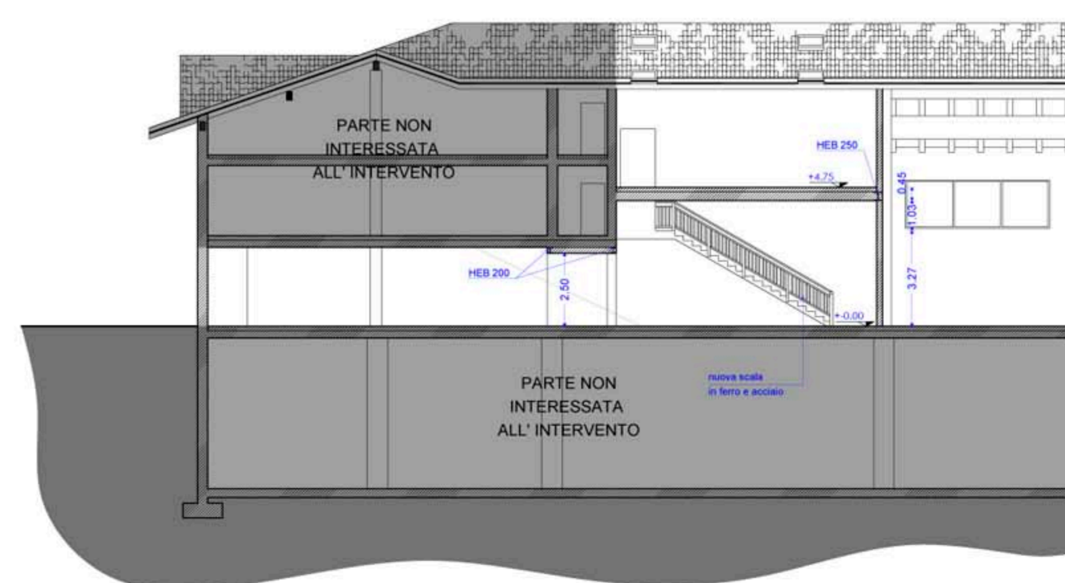
SEZIONE B-B
