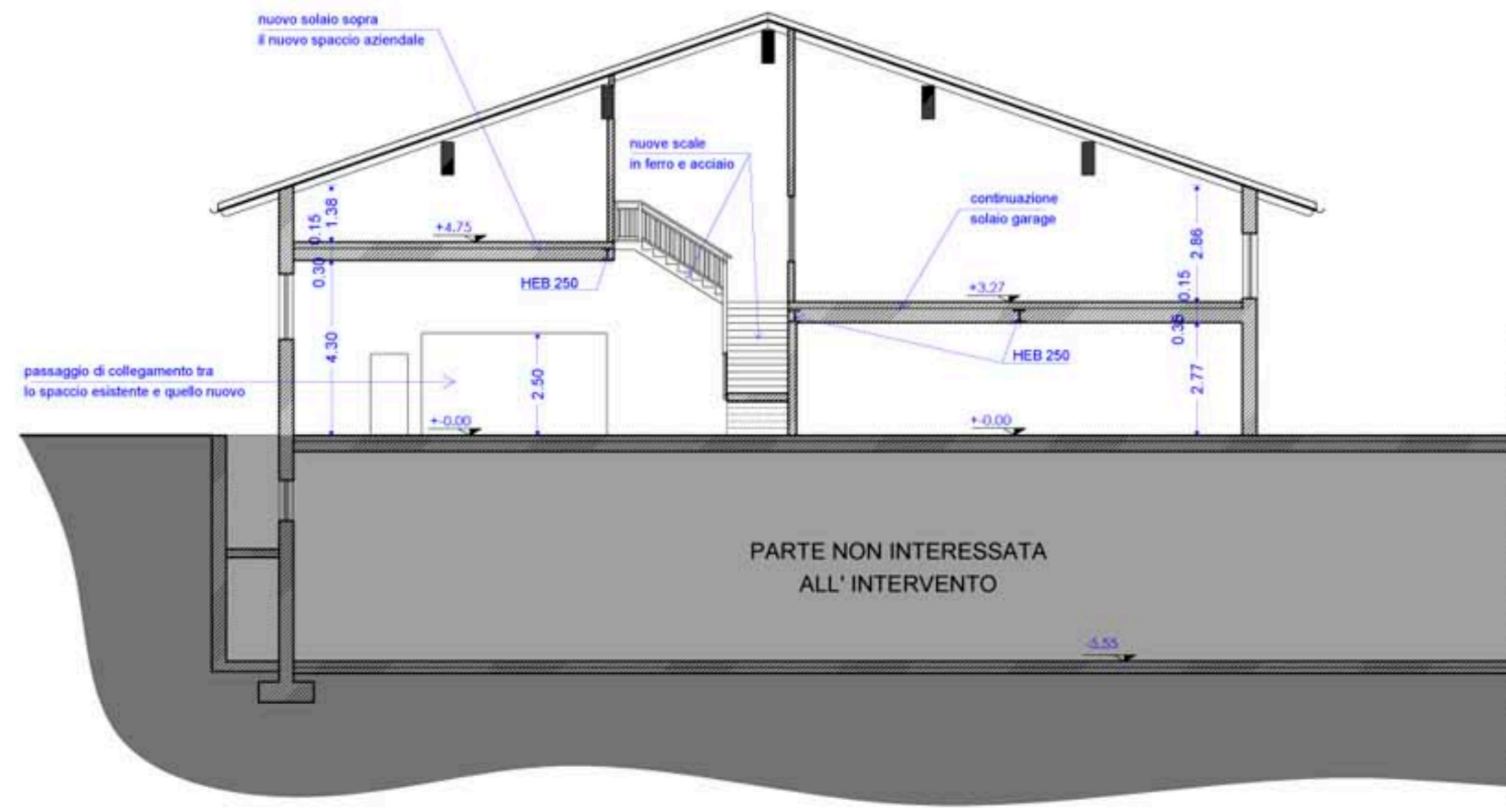
SEZIONE A-A
